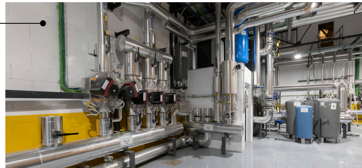
TECHNOTRAF Instal·lació d'autoconsum amb calderes de biomassa i refredadora d'absorció St. Vicenç de Torelló, Barcelona Superfície construïda: 9.500 m 2
